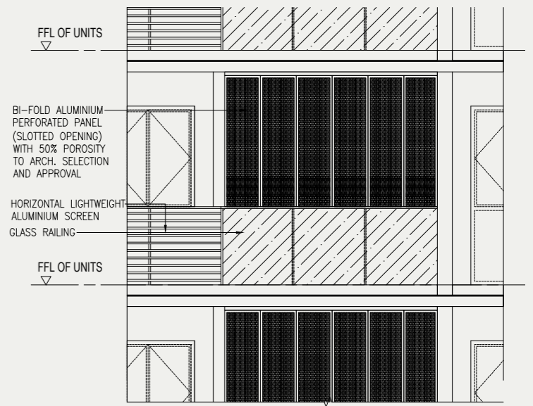
Elevation
